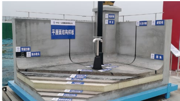
平屋面样板
