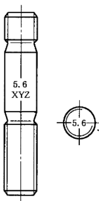
图 14 螺柱标志示例
