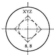
图 13 圆头方颈螺栓标志示例
