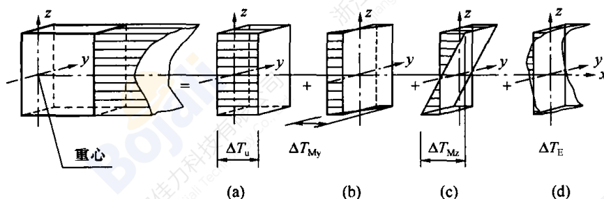
图 9 结构构件任意截面上的温度分布
