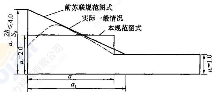
图 5 高低屋面处雪堆分布图示
