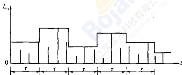
图 4 临时性活荷载随时间变化示意图
