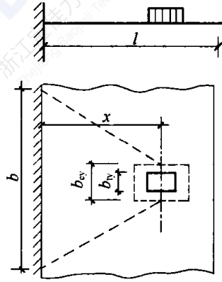
图 C. 0. 5-4 悬臂板上局部荷载的有效分布宽度
