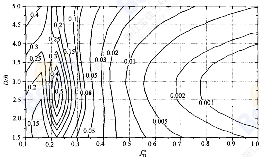
图 H. 3.4 扭矩谱能量因子
