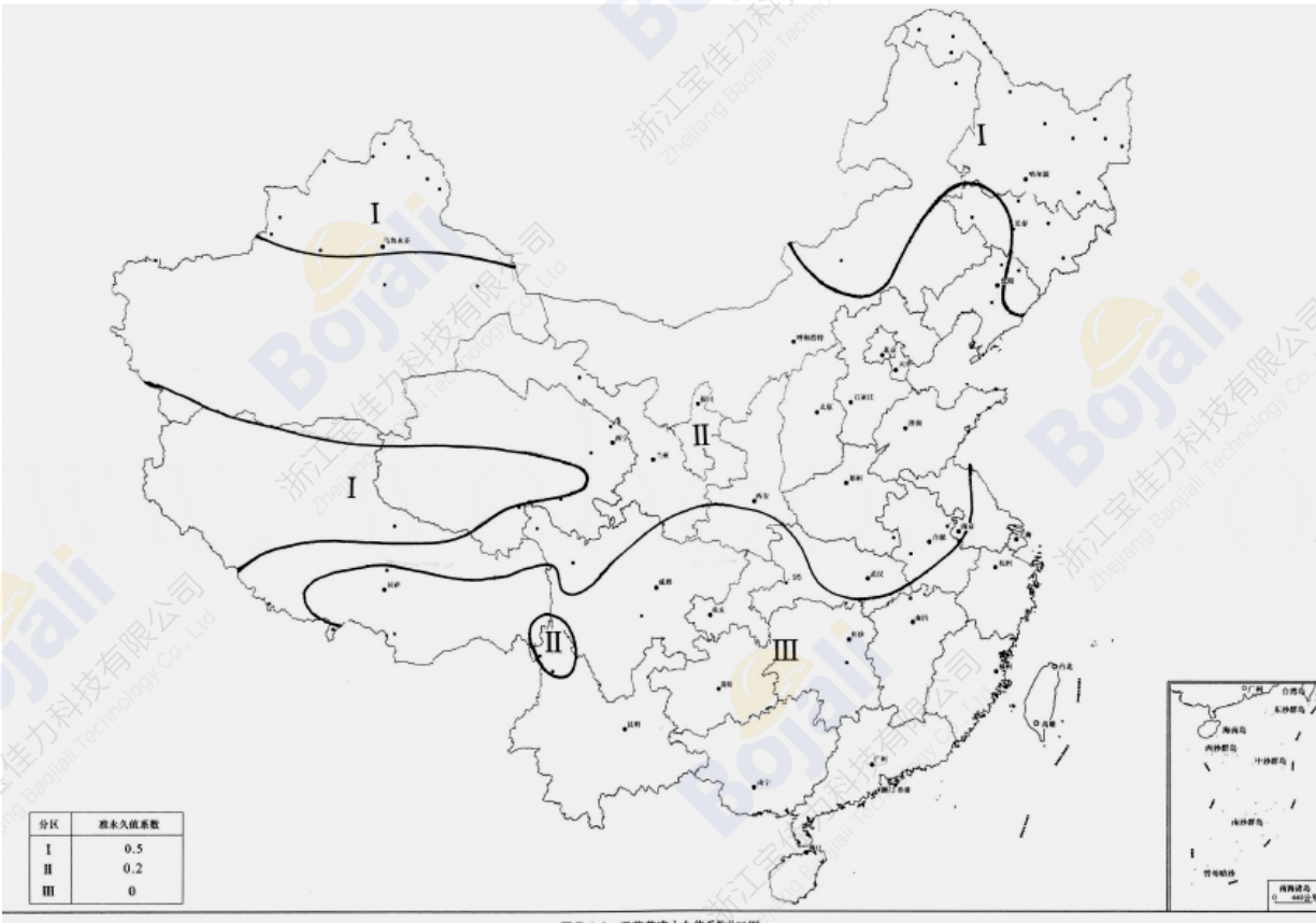
图 E.6.2 积雪荷载长期值分区图
