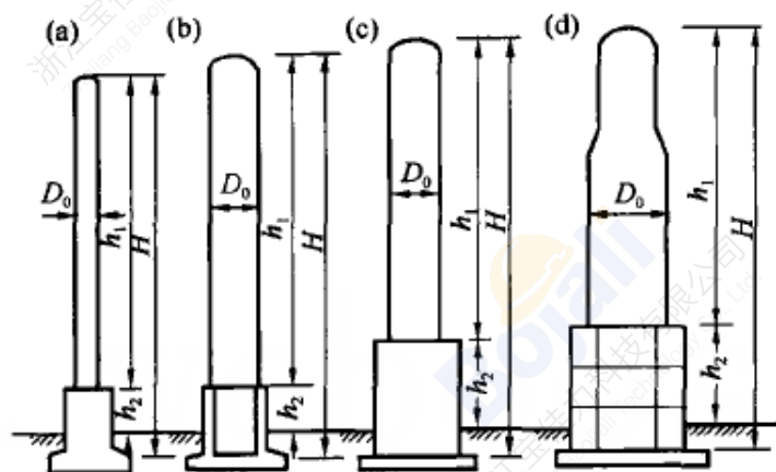
图 F. 1. 2 设备塔架的基础形式
