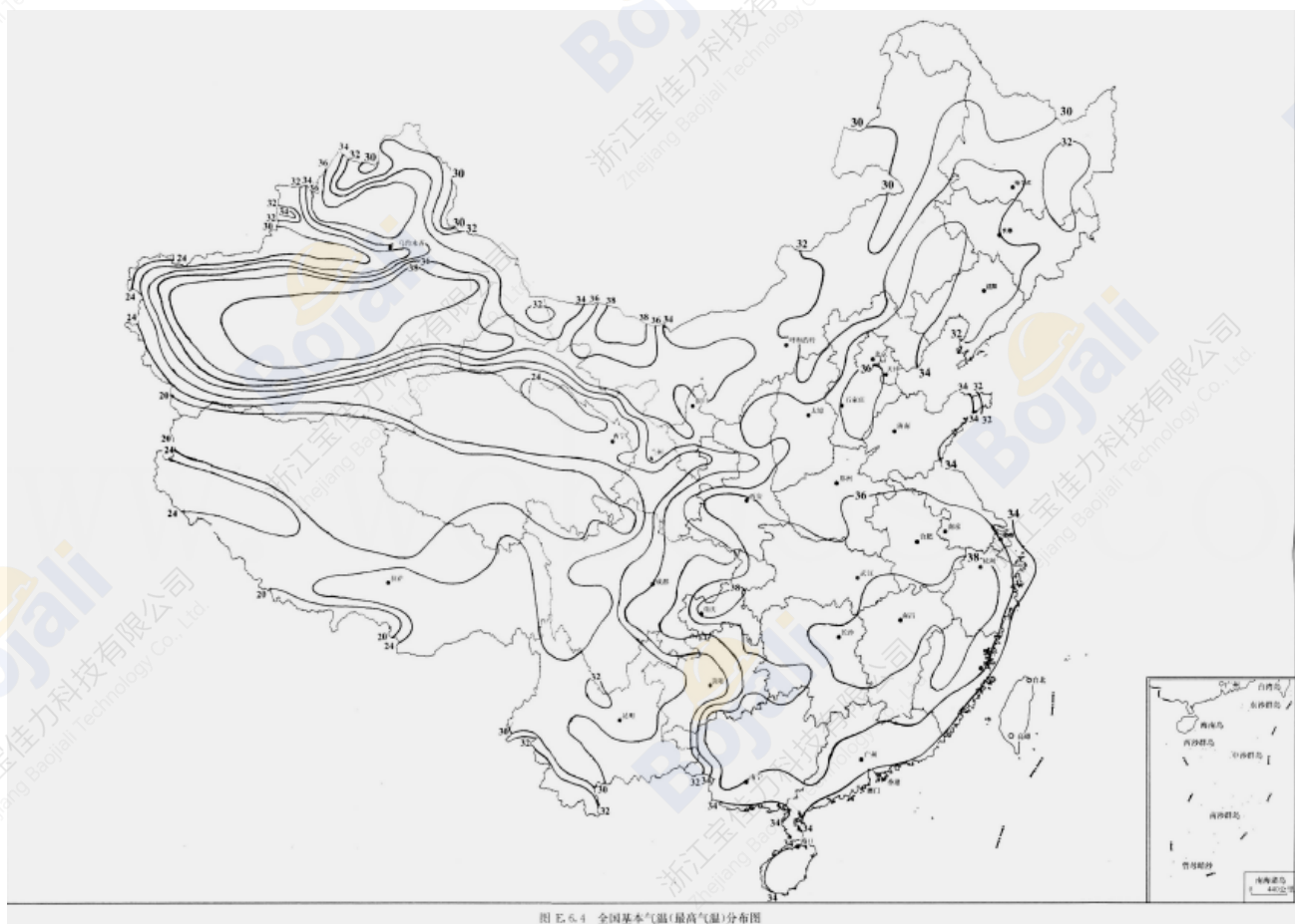
图 E.6.4 全国基本气温(最高气温)分布图
