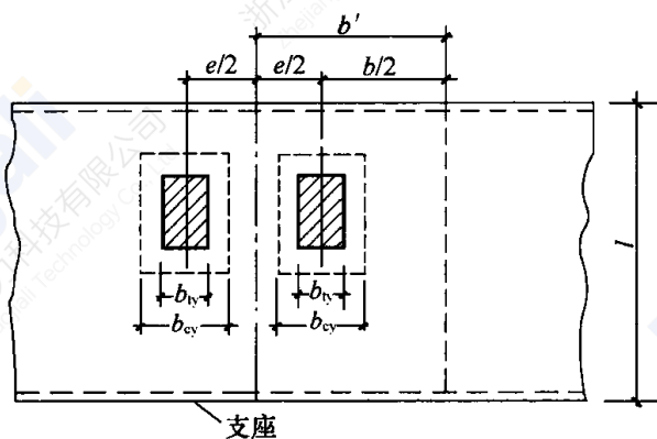
图 C.0.5-3 相邻两个局部荷载的有效分布宽度
