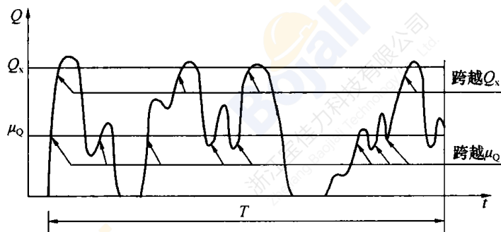
图 2 可变荷载按跨阈率确定代表值示意图
