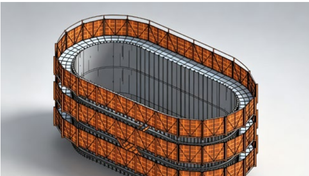
墩身模板一体作业平台
