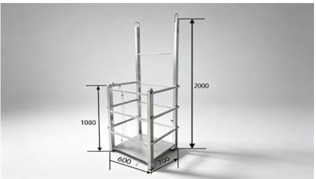
湿接缝吊篮
