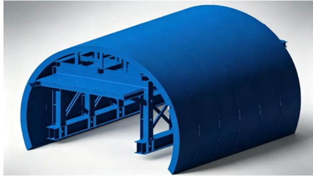
斜井二衬台车
