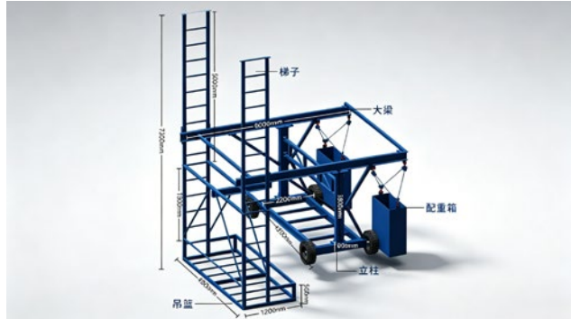
盖梁二次张拉台车
