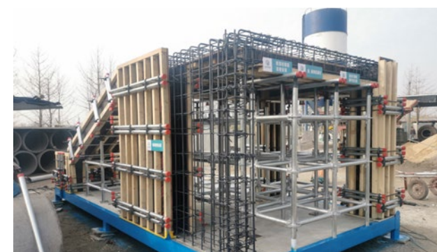
木工综合质量样板
