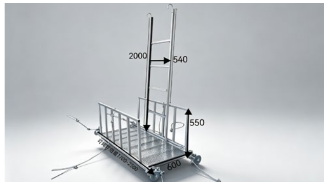
湿接缝张拉吊篮
