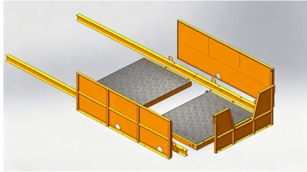
全拆卸式卸料平台
