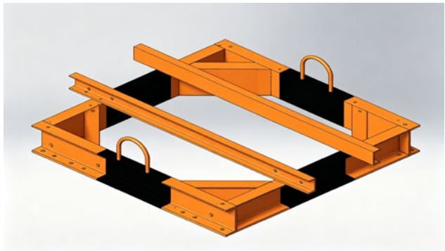
桩基固定钢筋笼扁担梁
